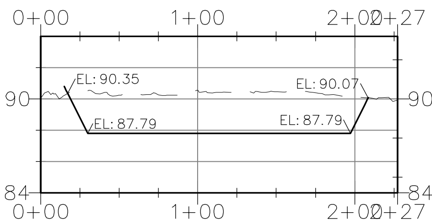
SECTION DD
